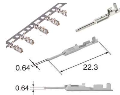
Terminal | 端子
