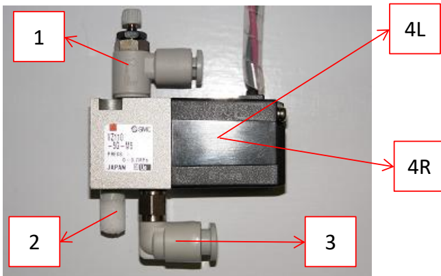
ロールアップ用ソレノイド (左/右) ソレノイドの加工以外同じ
